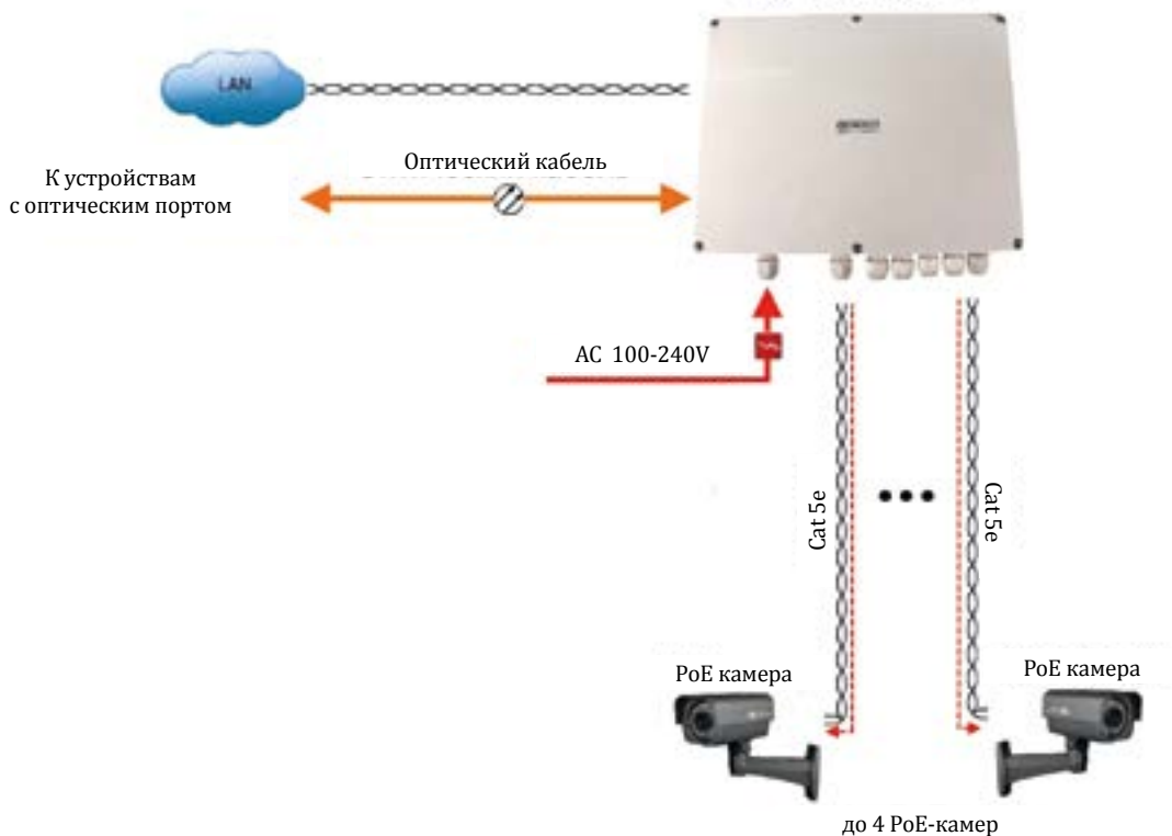
SW-40501/WC
