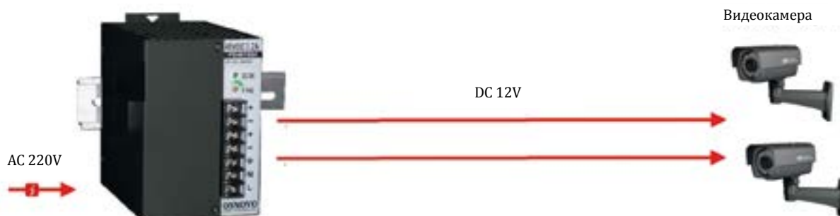
PS-12240/I
