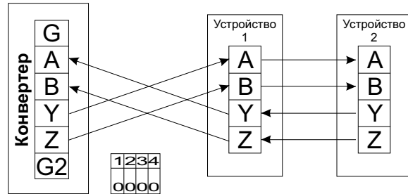
Схема подключения устройств с интерфейсом RS-422.
