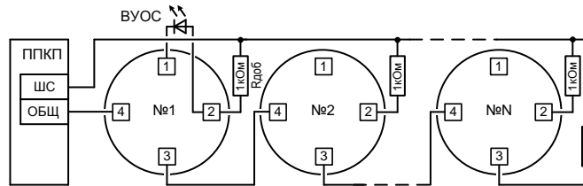
Рис.1 Типовая схема подключения извещателей к ППКП со знакопостоянным ШС. Величина резистора Rок определяется в соответствии с техническим описанием ППКП. Добавочный резистор Rдоб устанавливается – 1 кОм.
