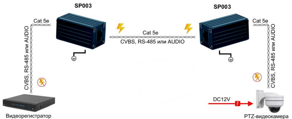
Рис.7 Схема подключения двухканального устройства грозозащиты SP003.
