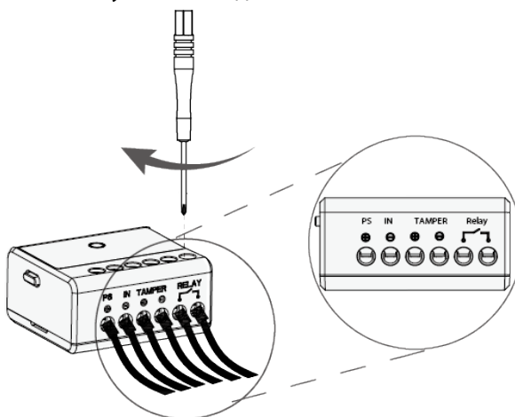
Рисунок 5-1 Подключение
