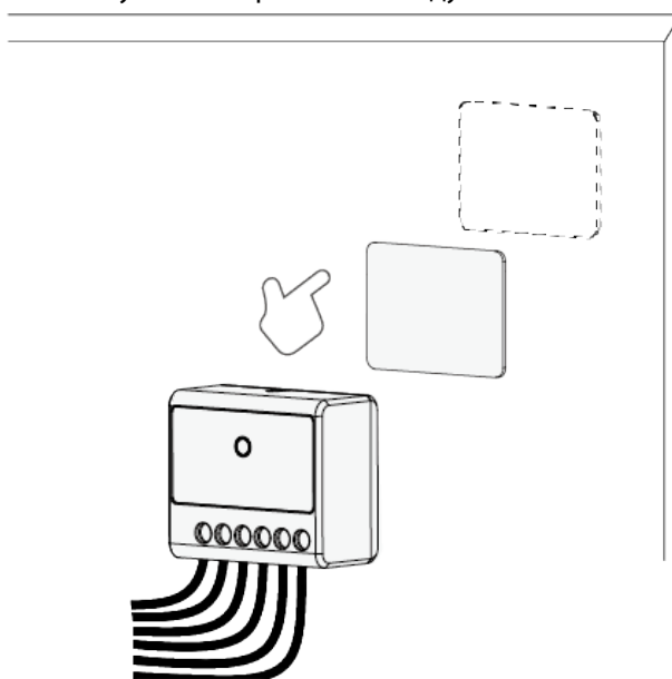
Рисунок 5-2 Крепление модуля
