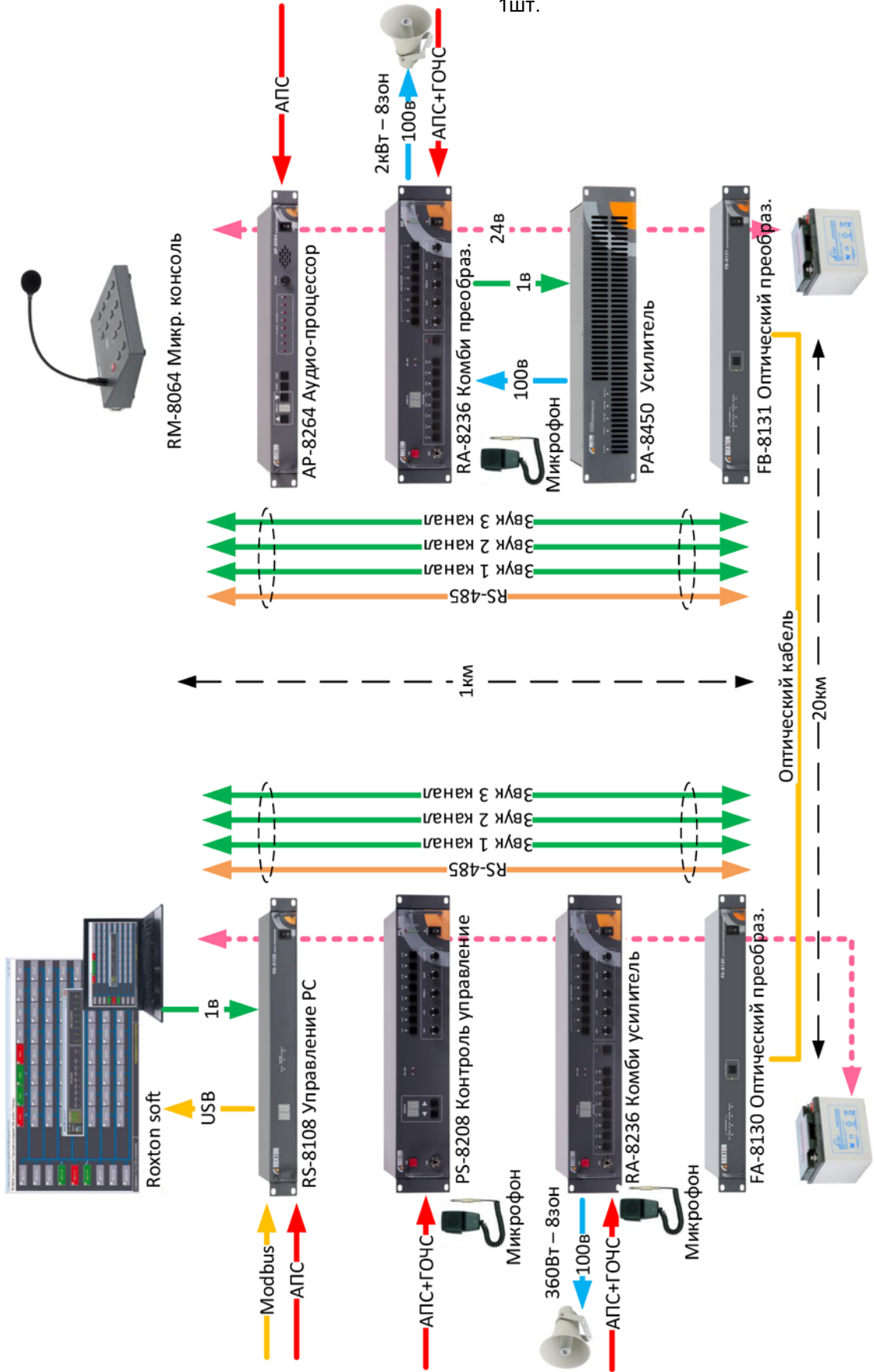
Функциональная схема системы оповещения ROXTON 8000
