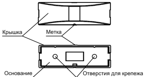
Рис.3 Конструкция магнита
