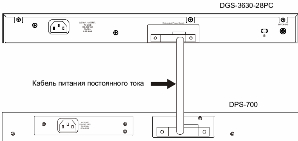
Рисунок 5 — Подключение DPS-700 к коммутатору
