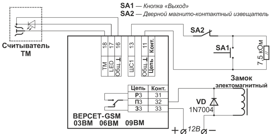
Рис.8. Схема организации Точки доступа.
